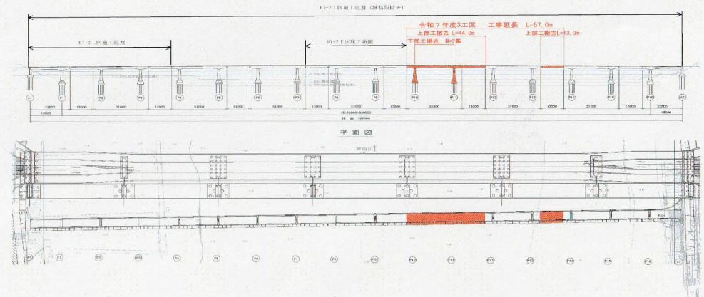
草戸大橋 上部工撤去工事 S=1:500 側 面 図
